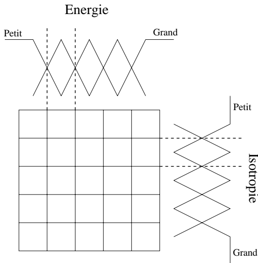
FIG. 3.: Principe de construction du tableau permettant l'acquisition des règles et des réglages des significations floues.
