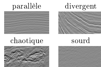
(b) Faciès sismiques
