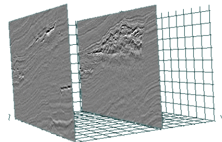
(a) Bloc sismique 3D
