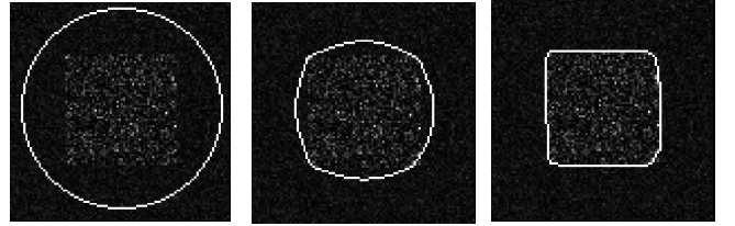
FIG. 1 : Evolution d'un contour actif sur une image de synthèse simulant deux régions K-distribuées.
